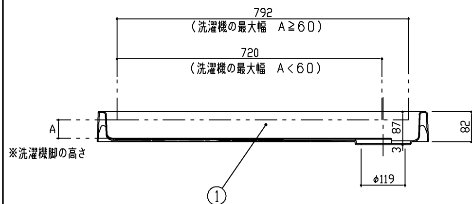
断面A-A
